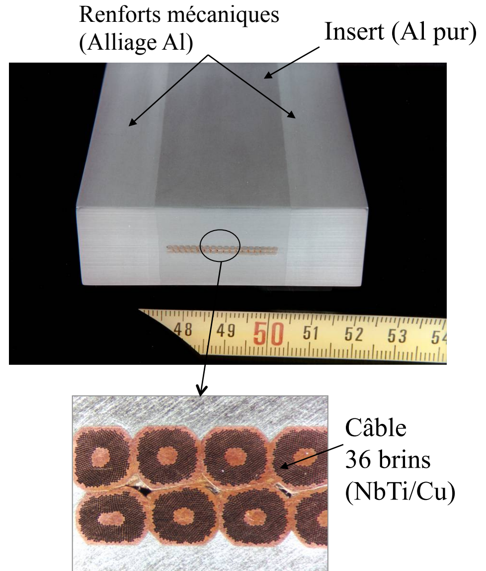
Conducteur CMS Solénoïde (T=4.2 K)
