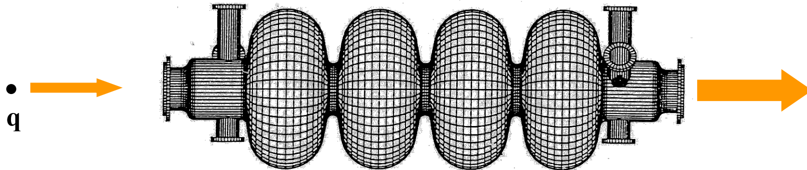
Cavité 4 cellules
