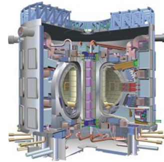
ITER (2025)
