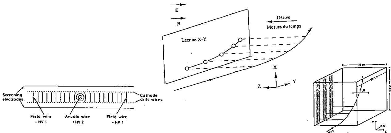
Figure 22 : gauche :localisation par temps de dérive dans une MWDC (Multi Wire Drift Chamber) ; milieu : principe de localisation 3D ; droite : application de ce principe à une TPC (Time Projection Chamber).
