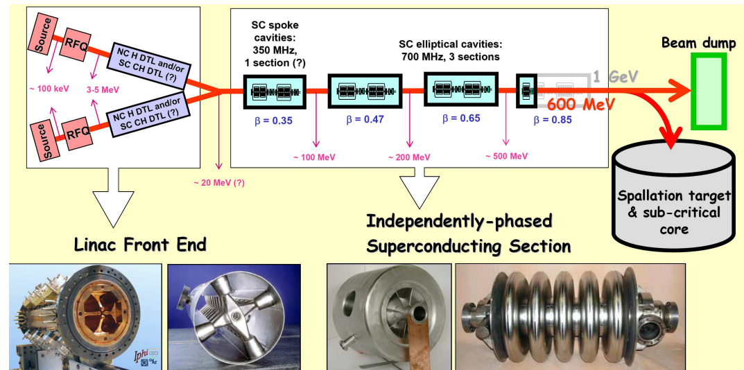
Conception du linac XT-ADS pour la transmutation des déchets nucléaires, axé sur la fiabilité
