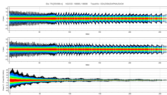
Conception du linac XT-ADS pour la transmutation des déchets nucléaires, axé sur la fiabilité
