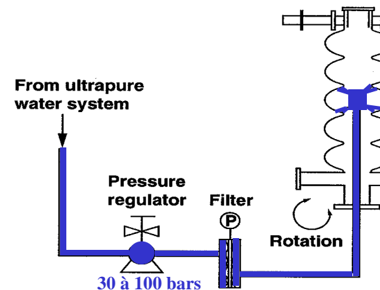
Système de rinçage à haute pression
