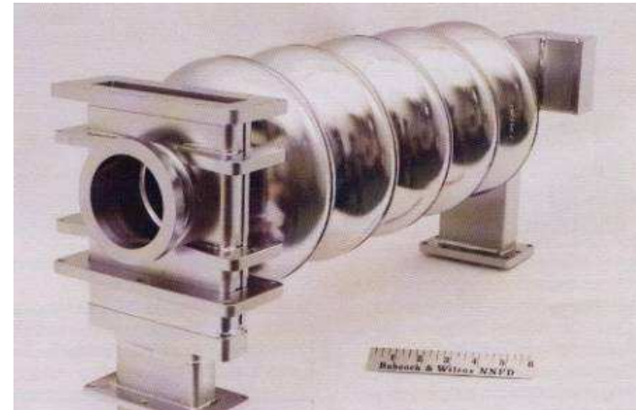
Cavité Nb 5 cellules – 1,5 GHz – 0,5m (Cornell → CEBAF)
