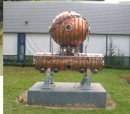
Cavités LEP1(CERN), 352 MHz -> accélération
