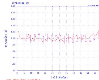
E_o/E_{design}
