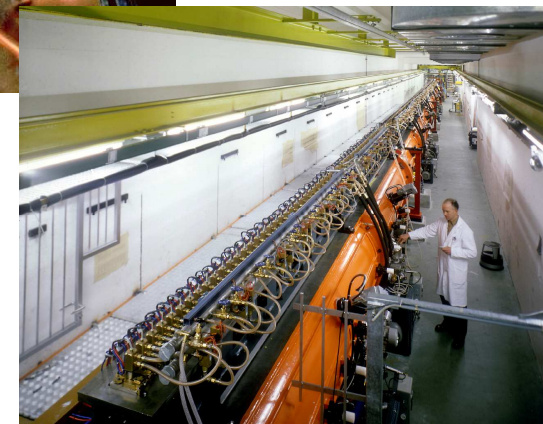
DTL Linac 2, (CERN, 1978) : 202 MHz, p 50 MeV
