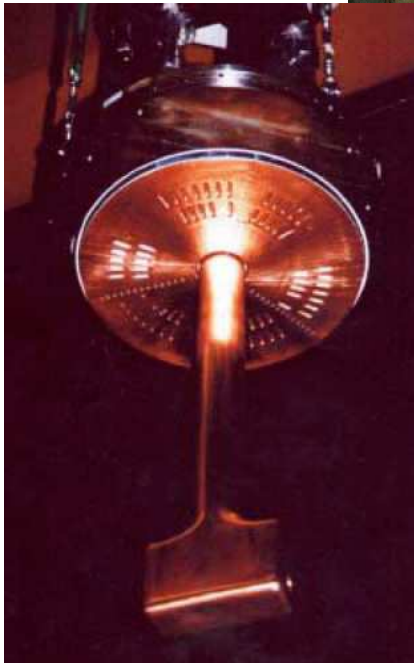
Regroupeur type quart d'onde (GANIL), 24 – 60 MHz
