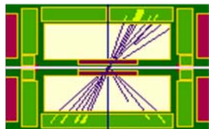
Événement hadronique
