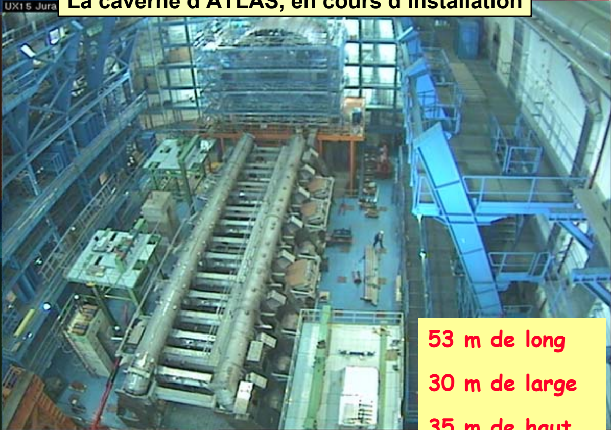
UX15 Jura La caverne d'ATLAS, en cours d'installation
