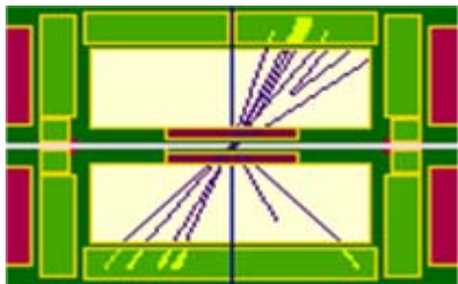
Evt Z^0 : beaucoup de particules et région centrale
