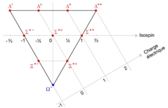
Découplet des baryons de spin 3/2.
