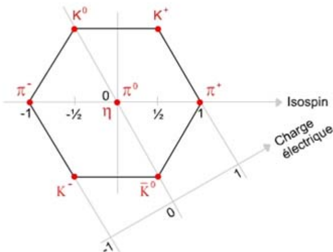
Découplet des baryons de spin 1/2.
